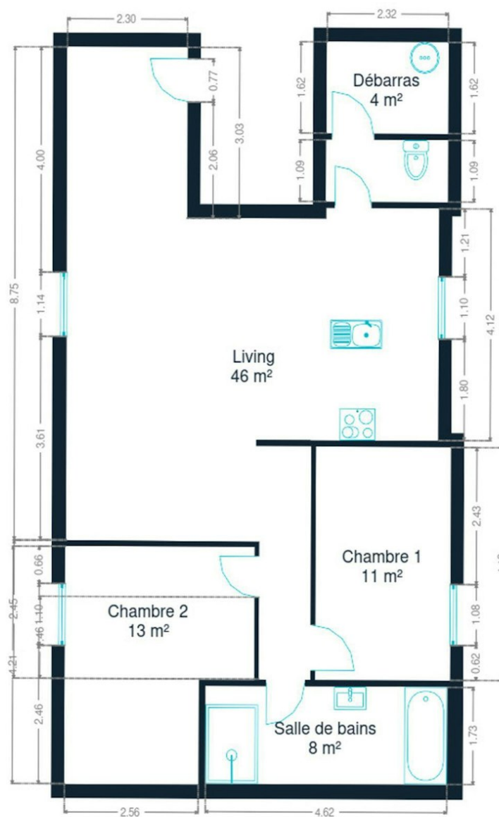
3ème étage
